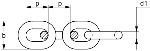
DIN 766
