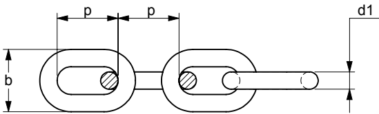
DIN 764
